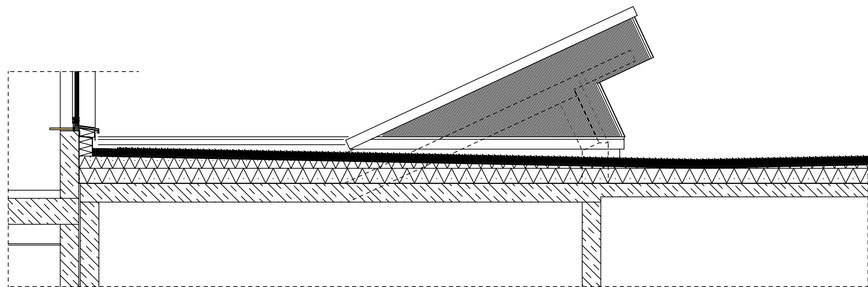
Schnitt H1
