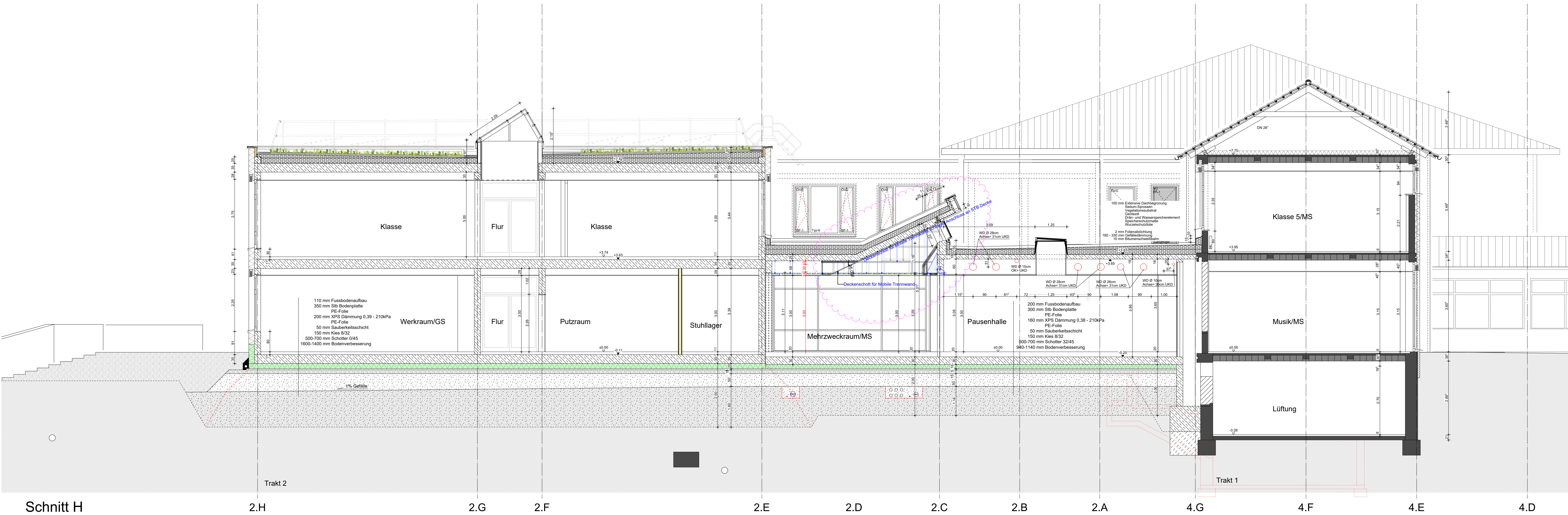
Schnitt H
